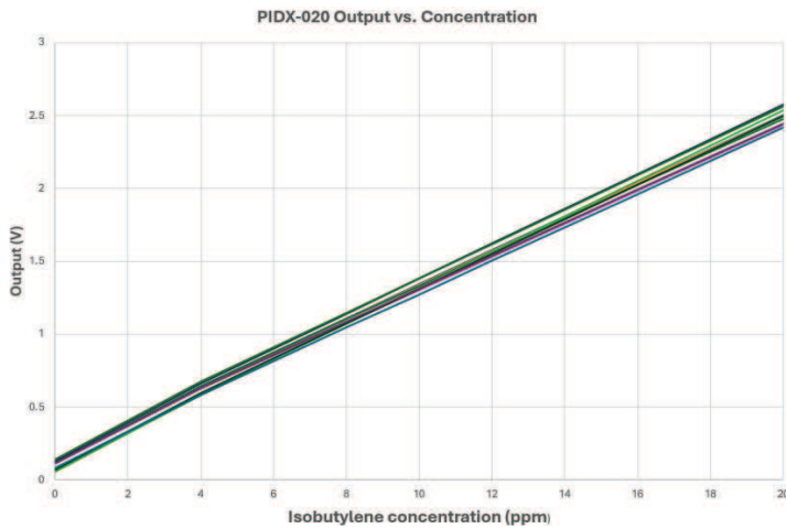
图1 PIDX-A-020 线性度 (0-20 ppm)
