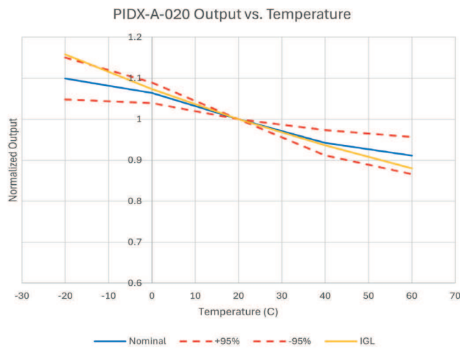
图2 灵敏度温度依赖性
