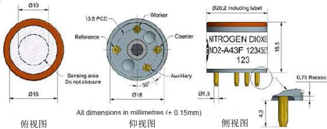
图1 NO2-A43F示意图
